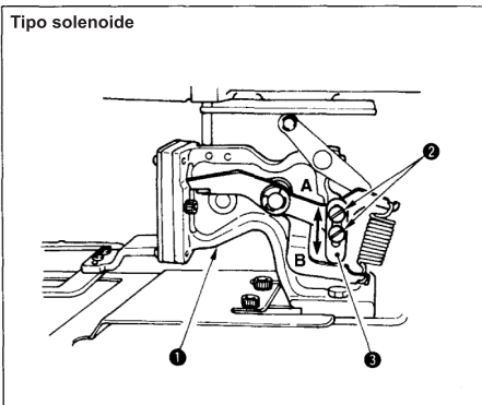
Tipo solenoide
